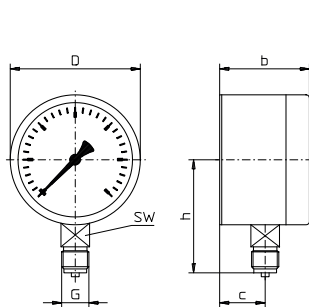
Typ R23.U.1.N... Anschluss unten bottom pressure entry raccord en bas
