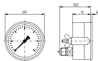
Typ R10.H.4.N... *) Dreieckfrontring triangular bezel collerette avant triangulaire
