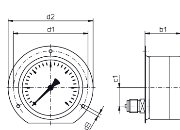
Typ R10.H.3.N... Rand hinten surface mounting flange rebord arrière
