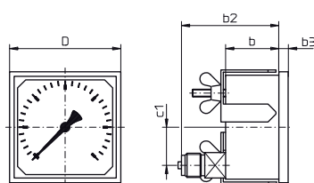
Typ R10.H.2.N... Quadratgehäuse DIN 43700 square panel mounting boîtier carré
