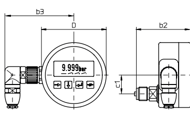
Typ ME15.H.1.N... Anschluss hinten back pressure entry raccord arrière
