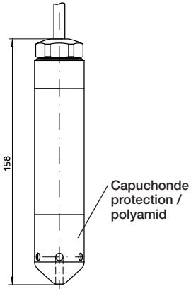
Sonde de puits
