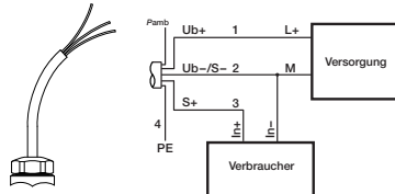
Kabelanschluss, 3-Leiter 0 ... 20 mA, 0 ... 10 V
