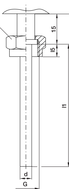
Form 5 Überwurfmutter union nut écrou chapeau
