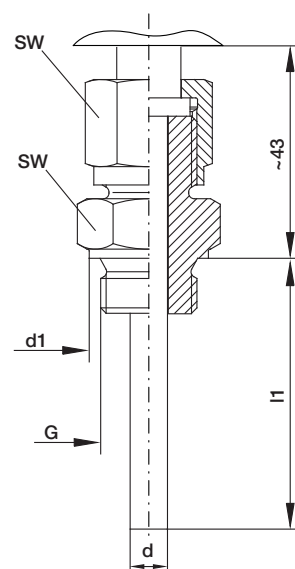
Form 9 Überwurfmutter mit Doppelnippel coupling nut with double nipple écrou avec double mamelon
